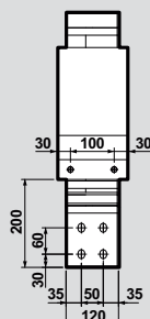
UB RCP 1250A AI
