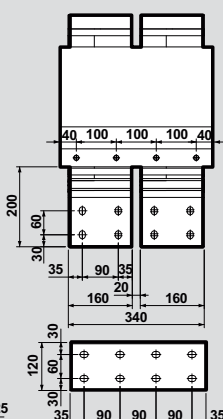
N. 2 FASES EN PARALELO
