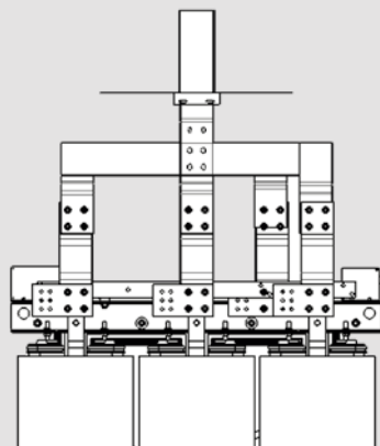
Transformador encapsulado en resina Zucchini
