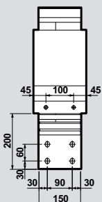
UB RCP 4000A AI
