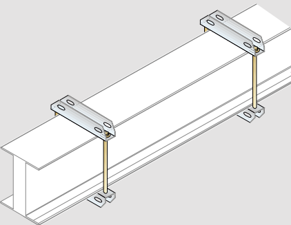
Horizontal en paralelo
