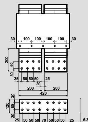
N. 2 FASES EN PARALELO
