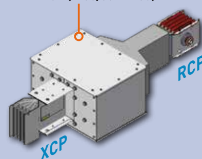
ADAPTADOR (IP55/65 A IP68)
